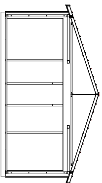
Coupe E-E
